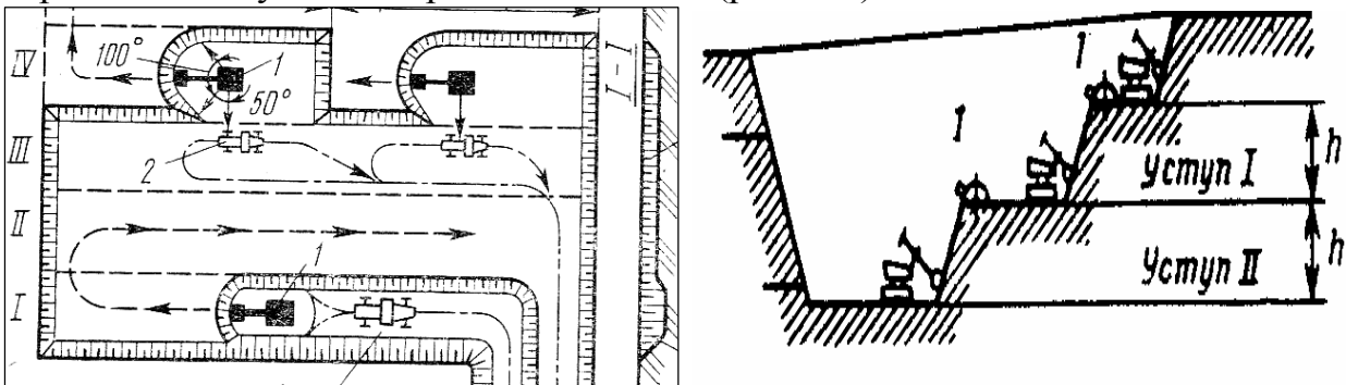
Рис. 2.1 - Схема розробки кар'єру землерійними машинами 1- екскаватор в забої; 2- автосамоскид.
