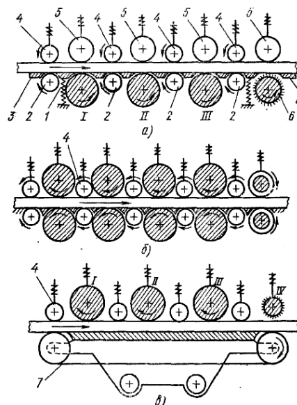
Рис. 3.10 - Схеми шліфувальних станків:
