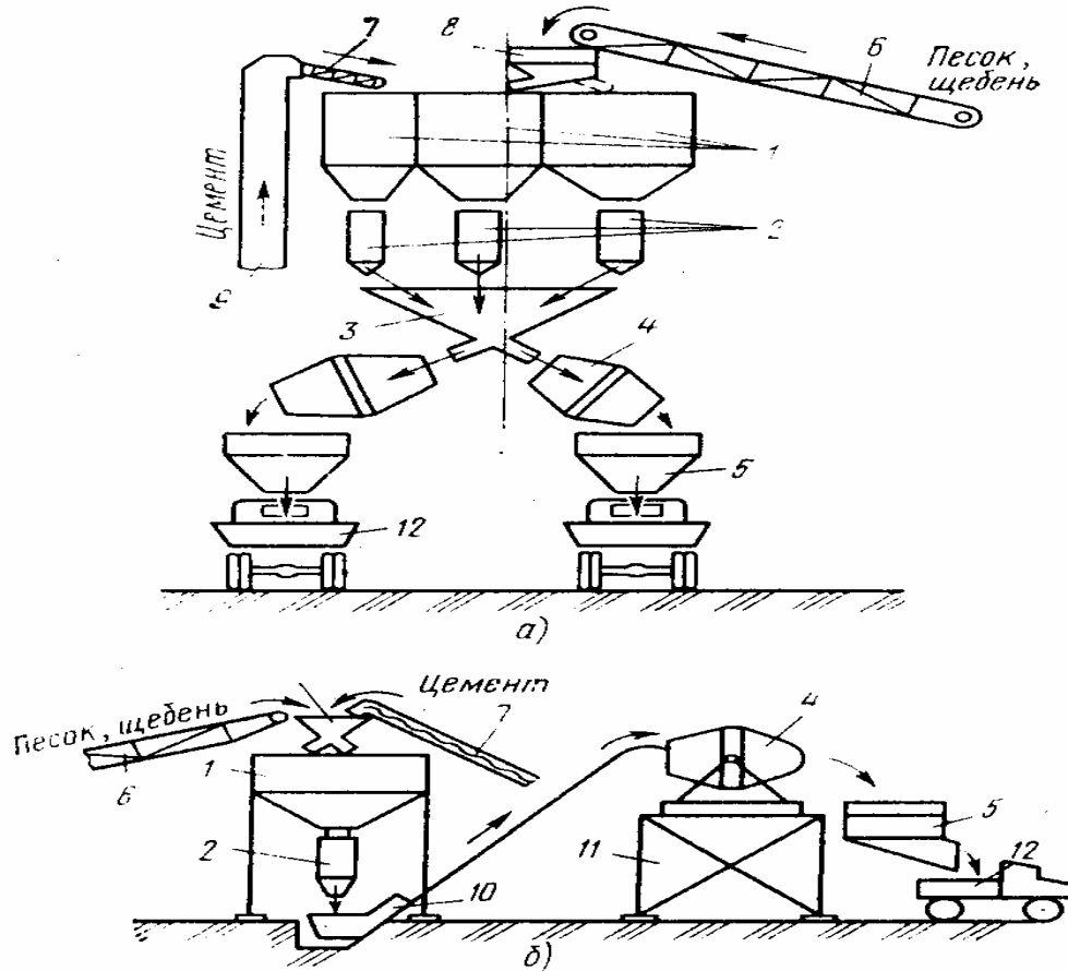
Рис. 2.5 – Схема компоновання технологічного обладнання бетонозмішувального підприємства:
