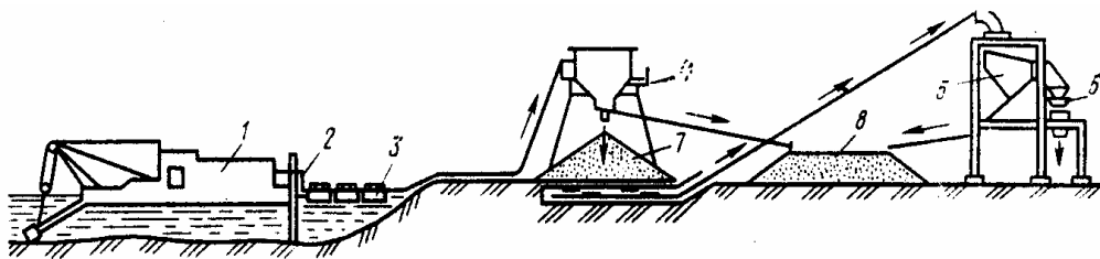
Рис. 2.3 – Схема видобування піску на гідро-механізованому кар'єрі : 1 – земснаряд, 2 – пульпопровід, 3 – понтони, 4, 5 – грохоти-класифікатори, 6 – конвеєр, 7 – карта наміву піску, 8 – склад гравію
