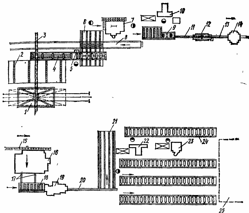
Рис. 3.8 – Схема потокової механізованої лінії виготовлення віконних плетень 1 - траверса; 2 - ланцюговий конвеєр; 3 - електроталь; 4, 15 - приводний роликовий конвеєр; 5 торцювальний верстат; 6, 21 - ланцюговий конвеєр; 7 - прирізний верстат; 8 - стрічковий конвеєр; 9 - автодатчик; 10 - свердлильний верстат; 11, 13, 20 - лотки; 12 - фугувальний верстат; 14 - рейсмусовий верстат; 16 - двосторонній шипорізний верстат; 17 - направляючі лінійки; 18 - приймально - передатний стіл; 19 - чотирибічний фрезерувально-кальовочний верстат; 22 – свердлильно - пазувальний верстат; 23 - фрезерний верстат; 24 - роликові столи; 25 - складальне відділення
