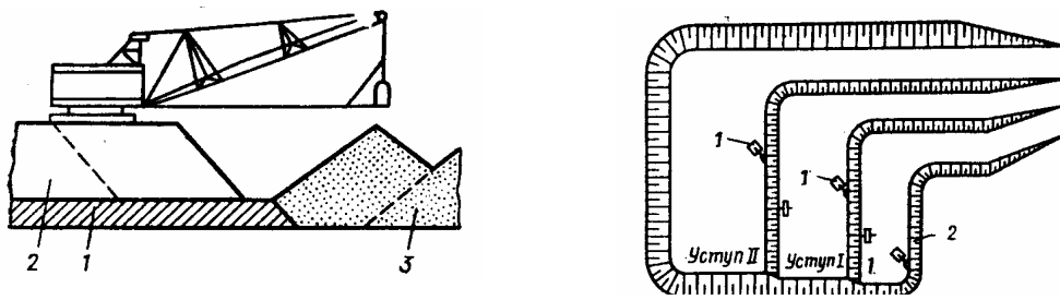
Рис. 2.2 – Безтранспортна схема розробки кар'єру драглайном: 1 – корисна порода; 2 – пуста порода; 3 – відвал
